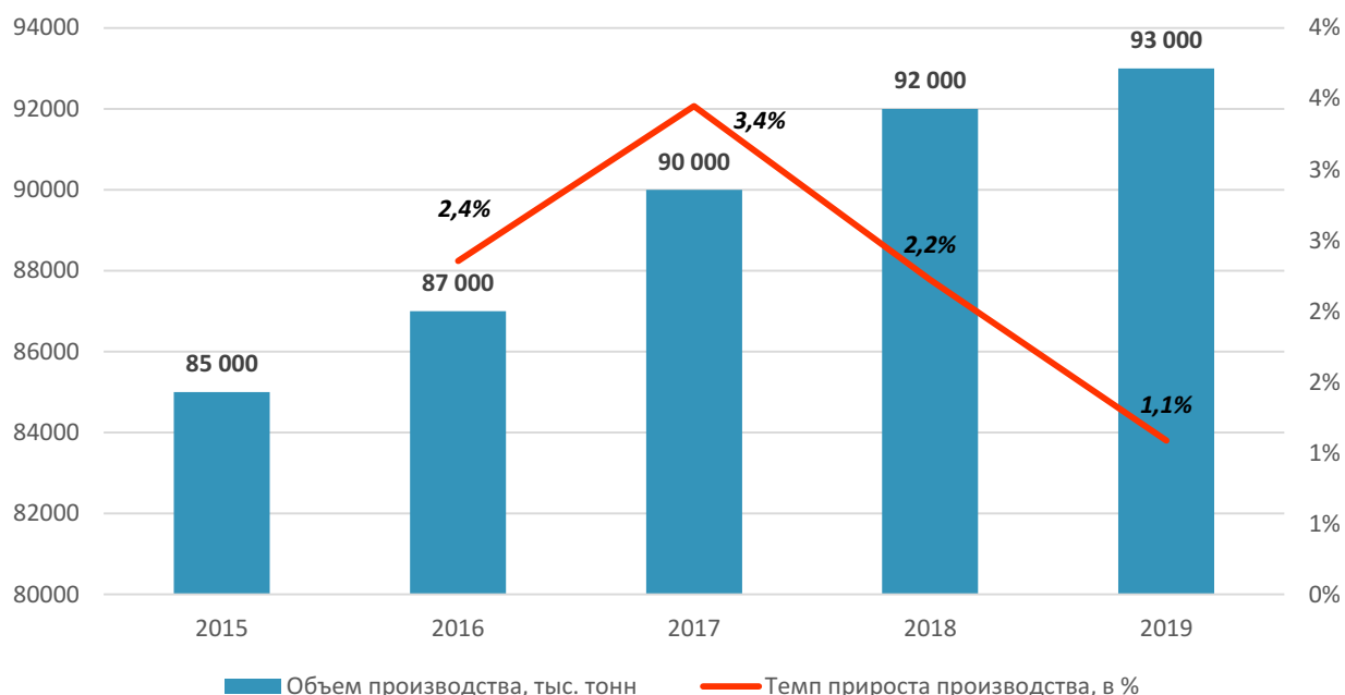
Диаграмма 11. Объем и темп прироста производства материалов для футеровки алюминиевых электролизеров (кремне-керамовермикулитовые плит) в России в 2015-2019 гг. в натуральном выражении, ..... и %.
