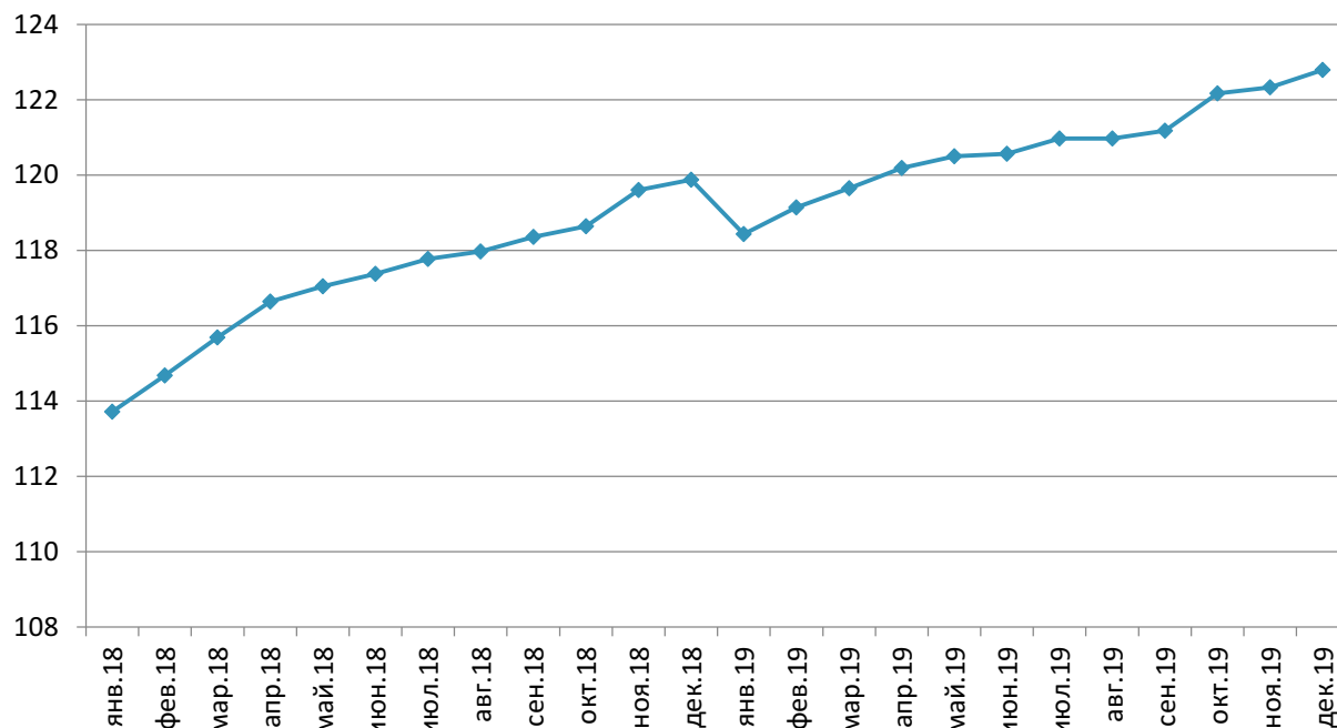
Диаграмма 21. Динамика средних цен на рынке мини-экскаваторов в России в 2018-2019 гг., руб.
