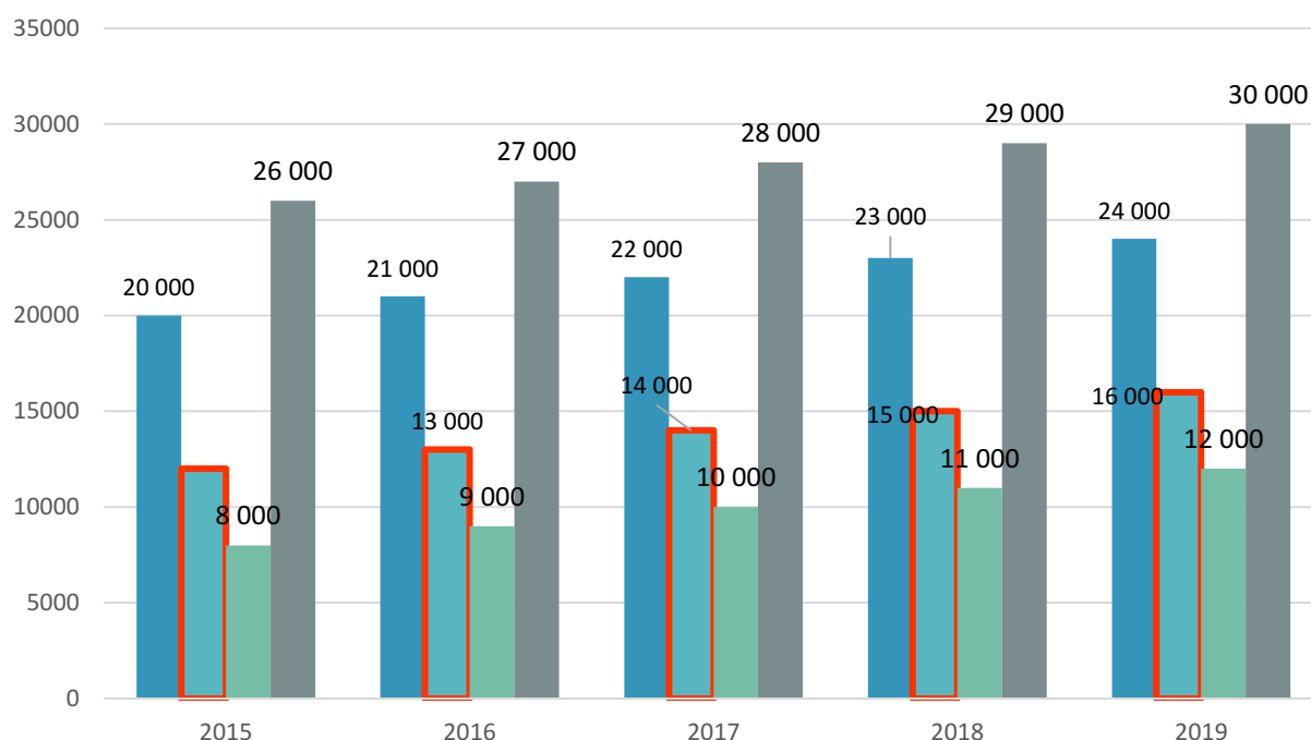
Диаграмма 5. Объём рынка оборудования для загрузки доменных печей в России по сегментам в 2015-2019 гг. в стоимостном выражении, $ тыс.
