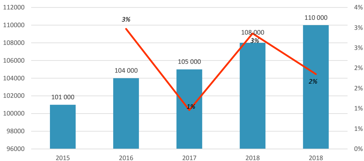
Диаграмма 1. Объем и темп прироста рынка оборудования для производства пружин в России в 2015-2019 гг. в натуральном выражении, ..... и %.
