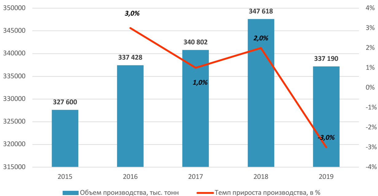
Диаграмма 12. Объем и темп прироста производства оборудования устьевого нефтяных и водозаборных скважин в России в 2015-2019 гг. в стоимостном выражении, $ тыс. и %.
