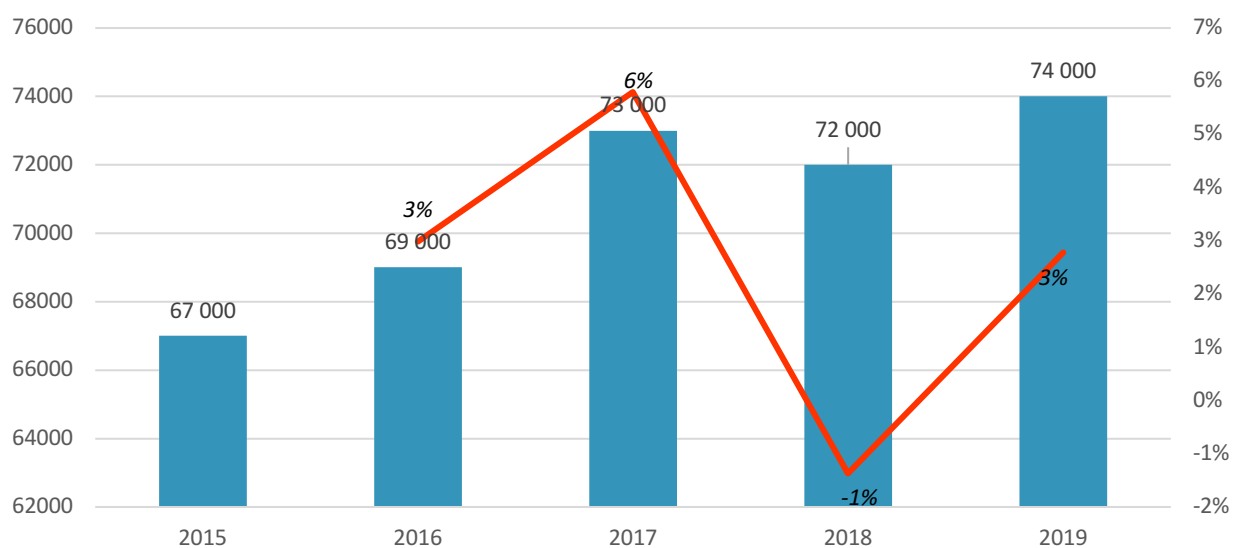
Диаграмма 16. Объём и темп прироста производства Сегмента 1 «.....» рынка оборудования формирования картонных коробок в России в 2015-2019 гг. в натуральном выражении, ..... и %.
