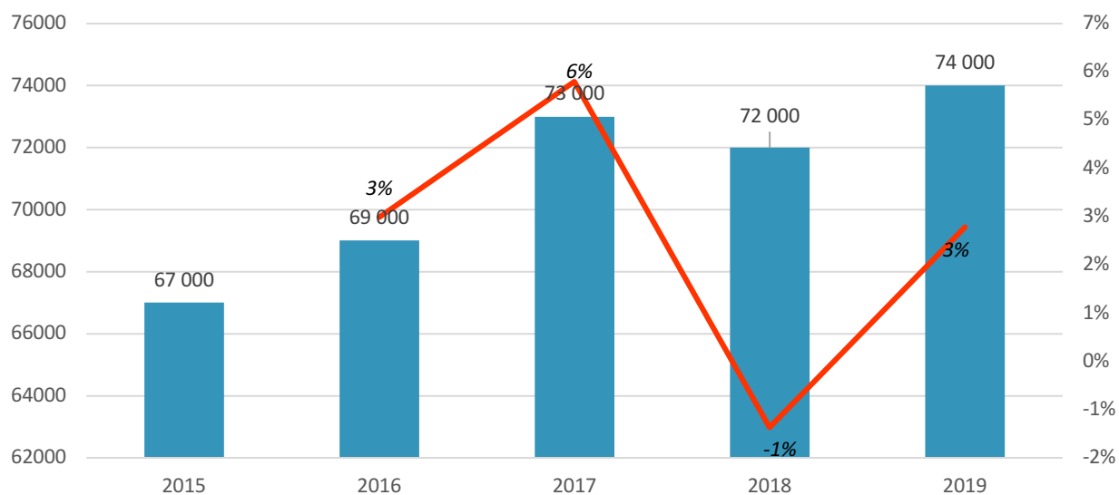
Диаграмма 16. Объём и темп прироста производства Сегмента 1 «.....» рынка опор (мачт) радиорелейных линий в России в 2015-2019 гг. в натуральном выражении, ..... и %.
