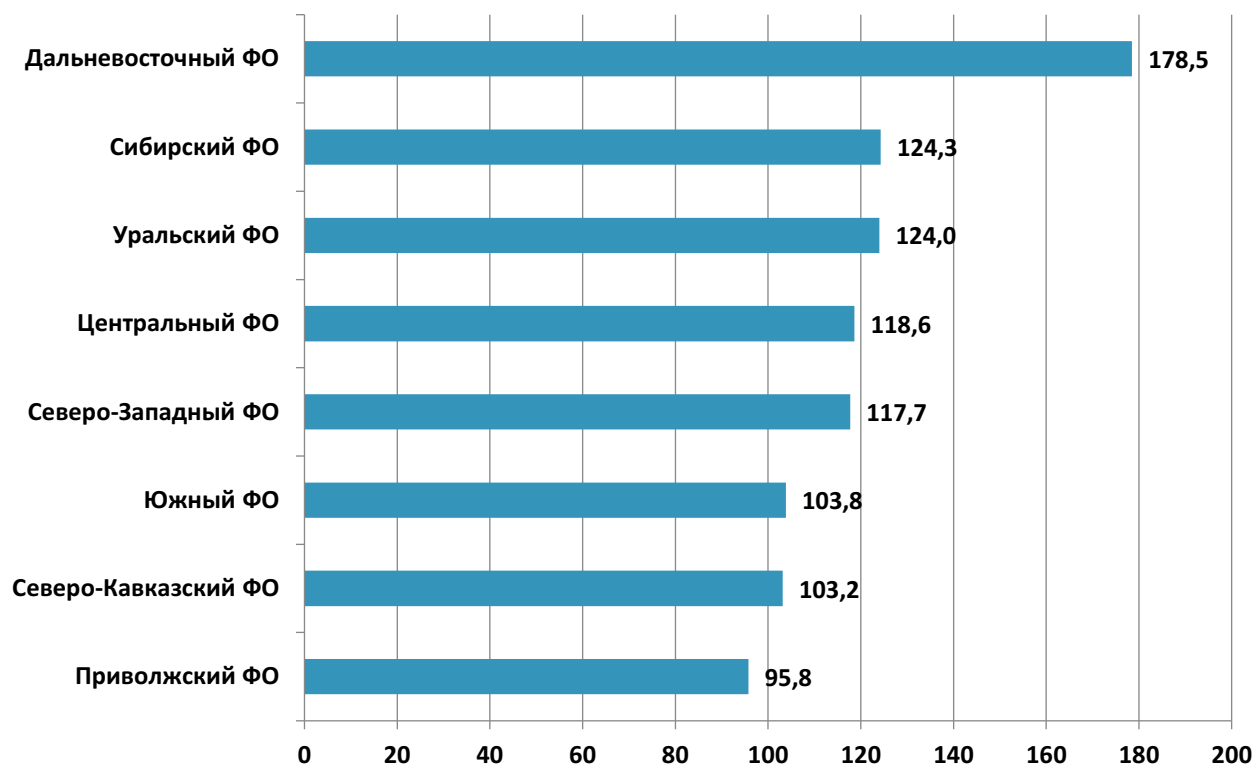
Диаграмма 20. Средние цены на рынке панелевозов по Федеральным Округам РФ в 2019 г., руб.
