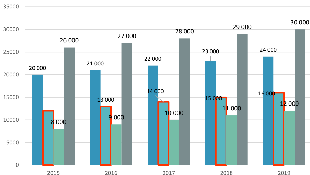
Диаграмма 3. Объем рынка панелевозов в России по сегментам в 2015-2019 гг. в натуральном выражении, .....
