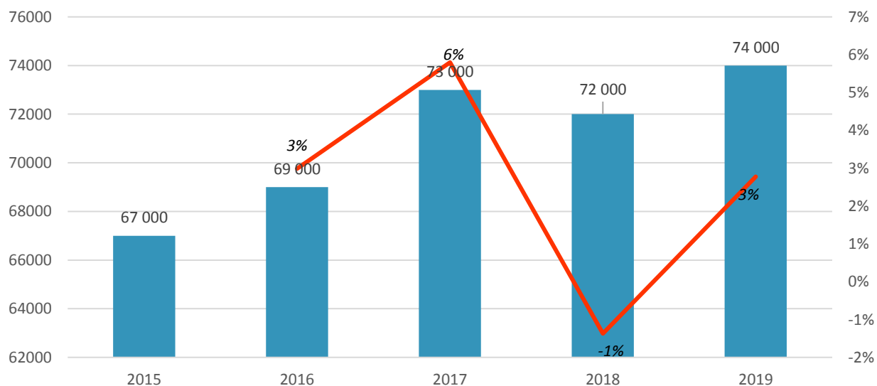
Диаграмма 16. Объём и темп прироста производства Сегмента 1 «.....» рынка приборов (устройств) электроизмерительных в России в 2015-2019 гг. в натуральном выражении, ..... и %.
