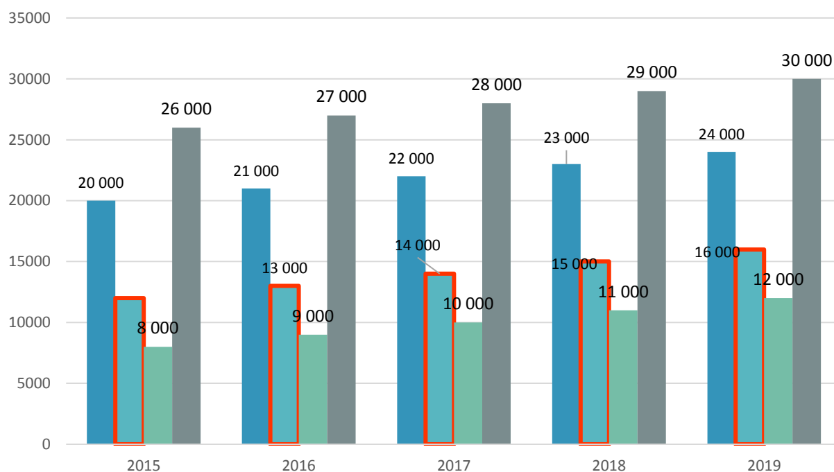
Диаграмма 5. Объём рынка приборов измерения индуктивности в России по сегментам в 2015-2019 гг. в стоимостном выражении, $ тыс.
