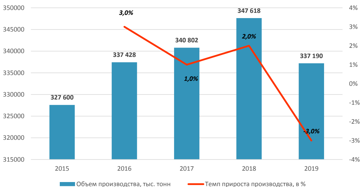
Диаграмма 12. Объем и темп прироста производства приборов измерения механических свойств материалов и линейных размеров в России в 2015-2019 гг. в стоимостном выражении, $ тыс. и %.
