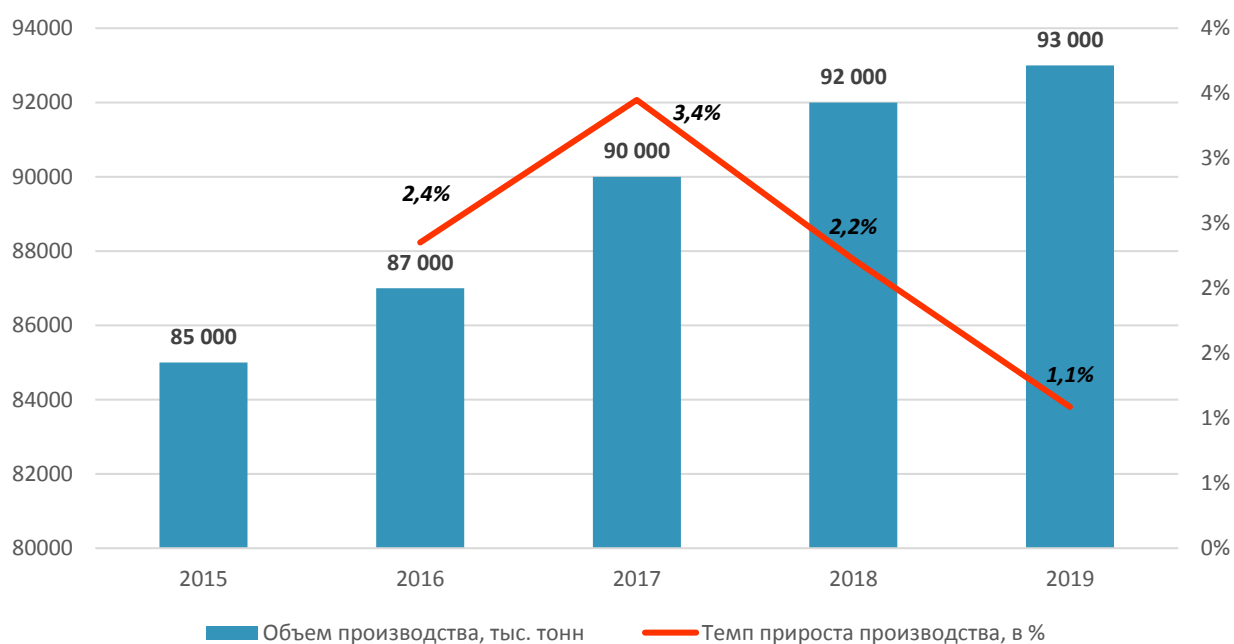
Диаграмма 11. Объем и темп прироста производства прицепов-цистерн и полуприцепов-цистерн для перевозки нефтепродуктов, воды и прочих жидкостей в России в 2015-2019 гг. в натуральном выражении, ..... и %.
