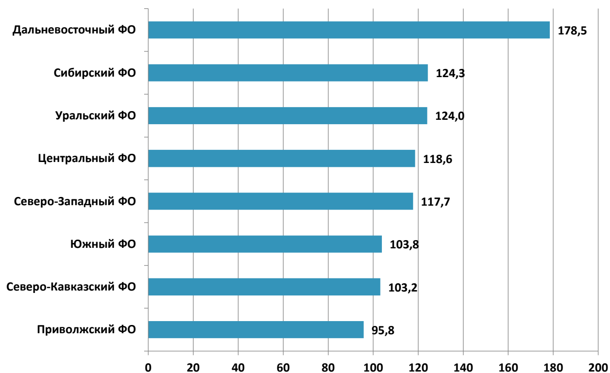
Диаграмма 20. Средние цены на рынке путей подкрановых по Федеральным Округам РФ в 2019 г., руб.
