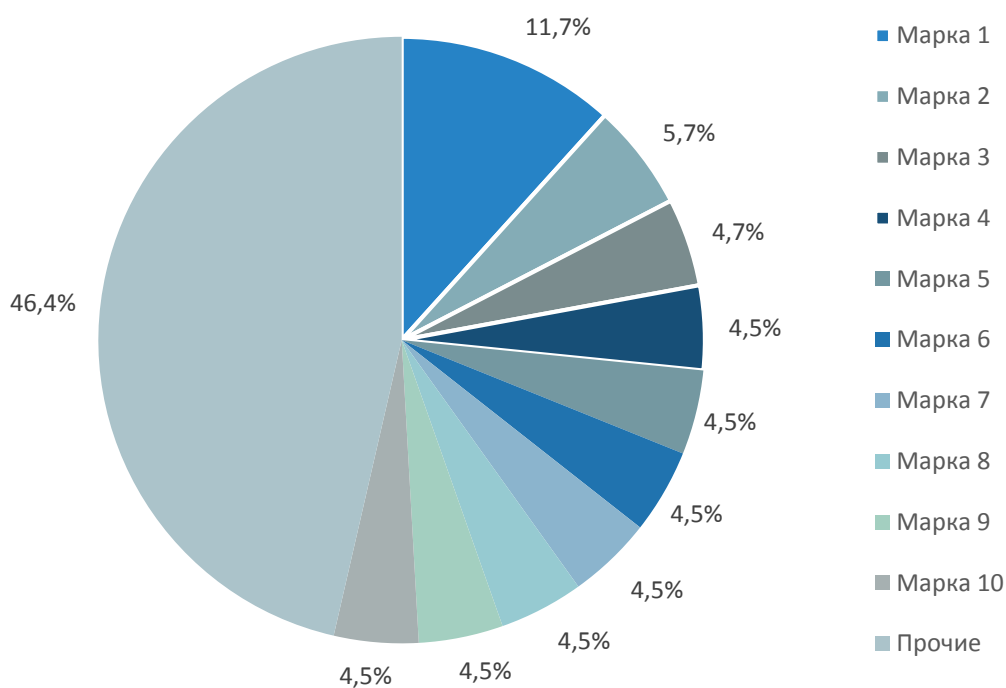
Диаграмма 8. Доли торговых марок в объеме рынка солидола в России в 2019 г., % от стоимостного объема.
