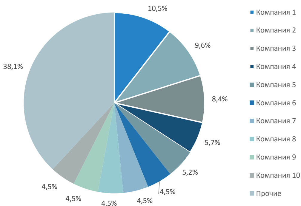
Диаграмма 7. Доли компаний в объеме рынка солидола в России в 2019 г., % от стоимостного объема.
