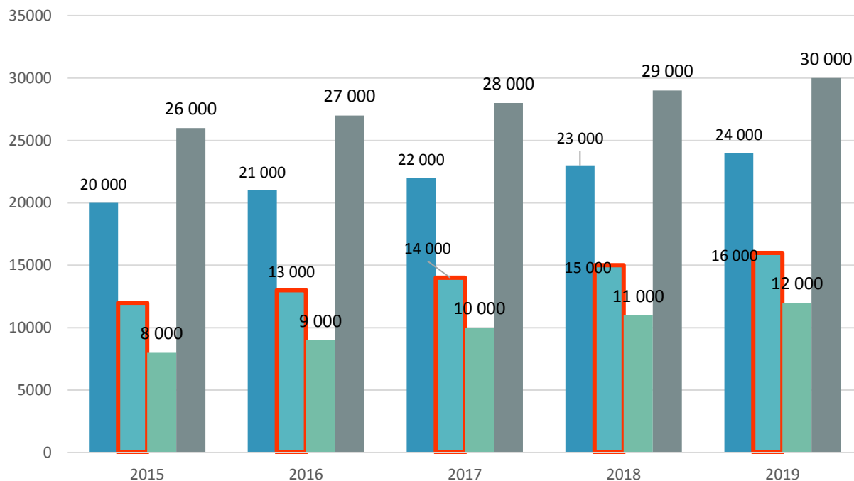
Диаграмма 5. Объем рынка станков болтонарезных в России по сегментам в 2015-2019 гг. в стоимостном выражении, $ тыс.
