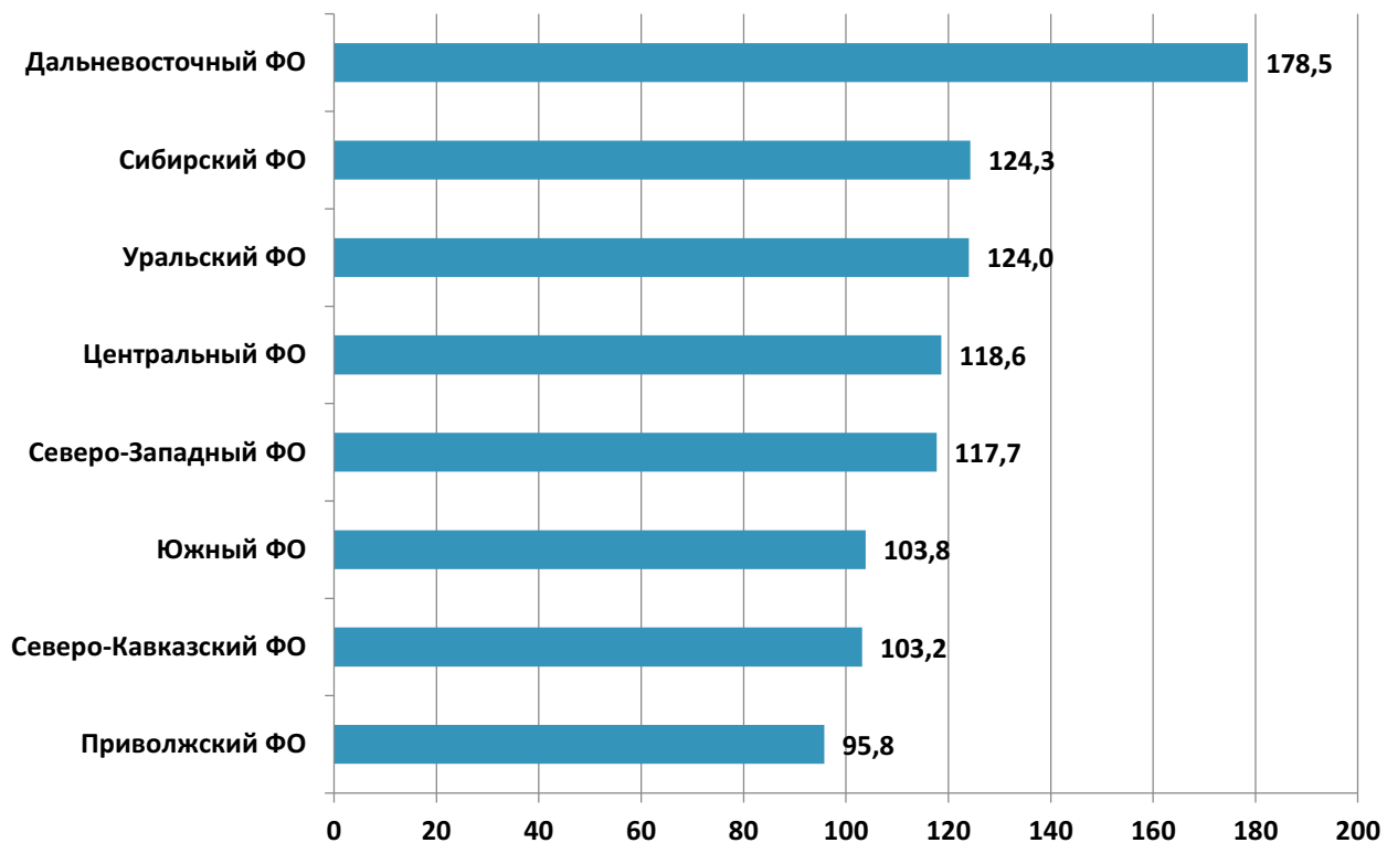
Диаграмма 20. Средние цены на рынке тестеров электрических по Федеральным Округам РФ в 2019 г., руб.
