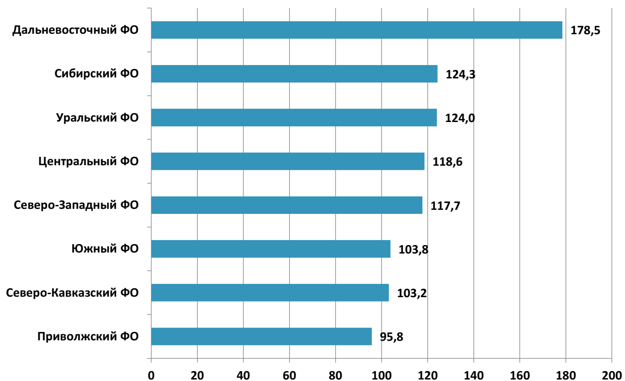
Диаграмма 20. Средние цены на рынке фильтров керамических по Федеральным Округам РФ в 2019 г., руб.
