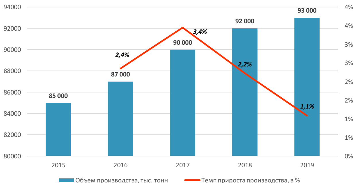
Диаграмма 11. Объем и темп прироста производства щебнераспределителей в России в 2015-2019 гг. в натуральном выражении, ..... и %.
