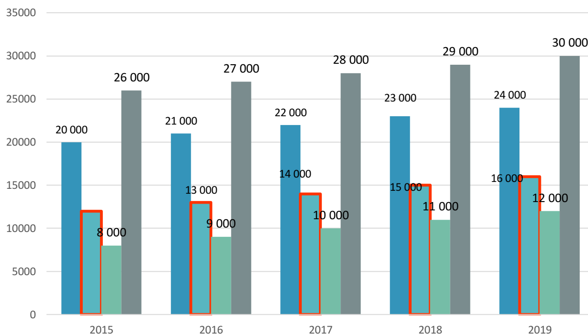
Диаграмма 3. Объем рынка щитов проходческих в России по сегментам в 2015-2019 гг. в натуральном выражении, .....
