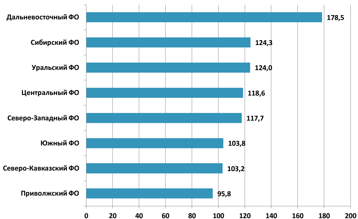
Диаграмма 20. Средние цены на рынке экскаваторов колесных по Федеральным Округам РФ в 2019 г., руб.
