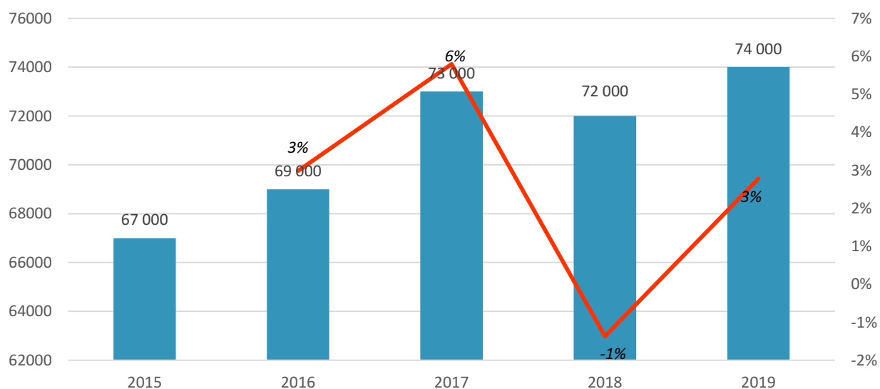
Диаграмма 16. Объём и темп прироста производства Сегмента 1 «.....» рынка систем приводных электромеханических в России в 2015-2019 гг. в натуральном выражении, ..... и %.
