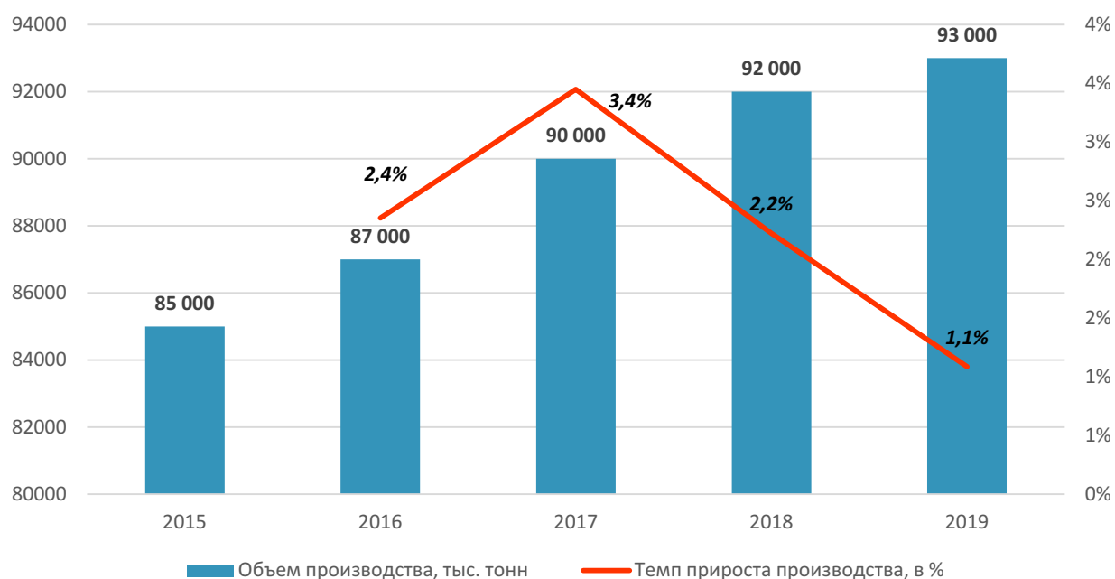
Диаграмма 11. Объем и темп прироста производства технологий гидроразрыва пласта в России в 2015-2019 гг. в натуральном выражении, ..... и %.
