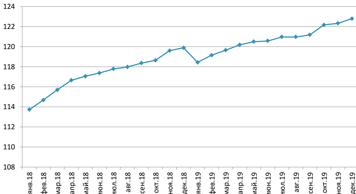
Диаграмма 21. Динамика средних цен на рынке генераторов рентгеновских в России в 2018-2019 гг., руб.
