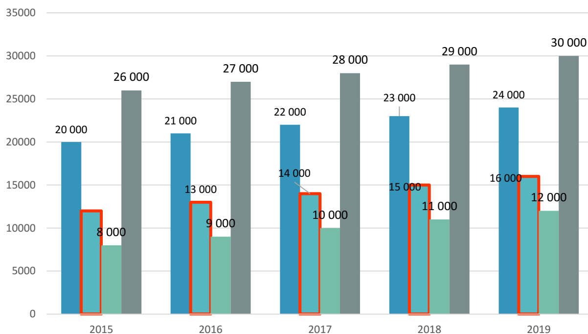
Диаграмма 5. Объем рынка дробилок валковых в России по сегментам в 2015-2019 гг. в стоимостном выражении, $ тыс.
