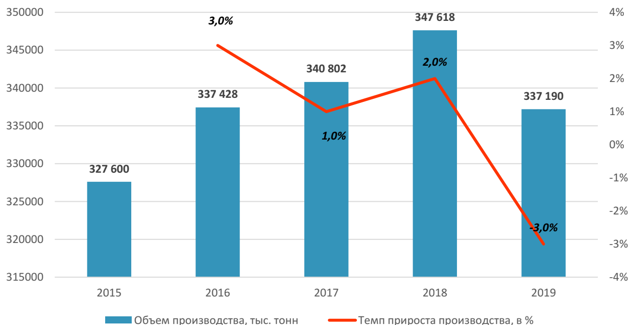
Диаграмма 12. Объем и темп прироста производства катков пневмоколесных в России в 2015-2019 гг. в стоимостном выражении, $ тыс. и %.
