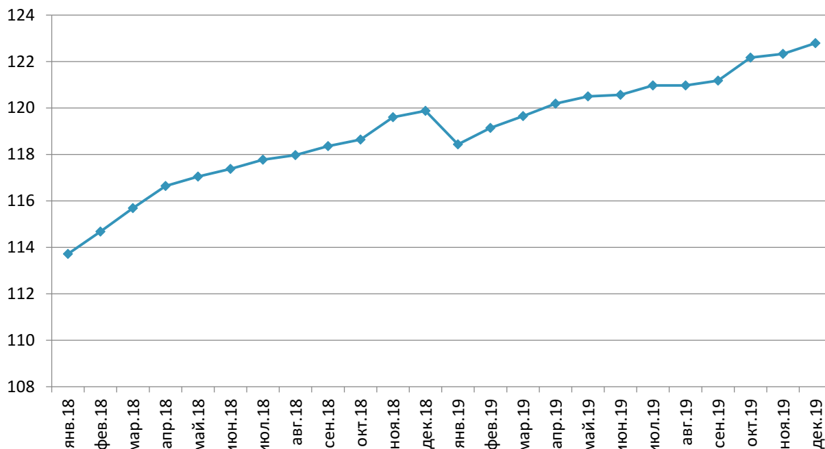
Диаграмма 21. Динамика средних цен на рынке клапанов-регуляторов уровня в России в 2018-2019 гг., руб.
