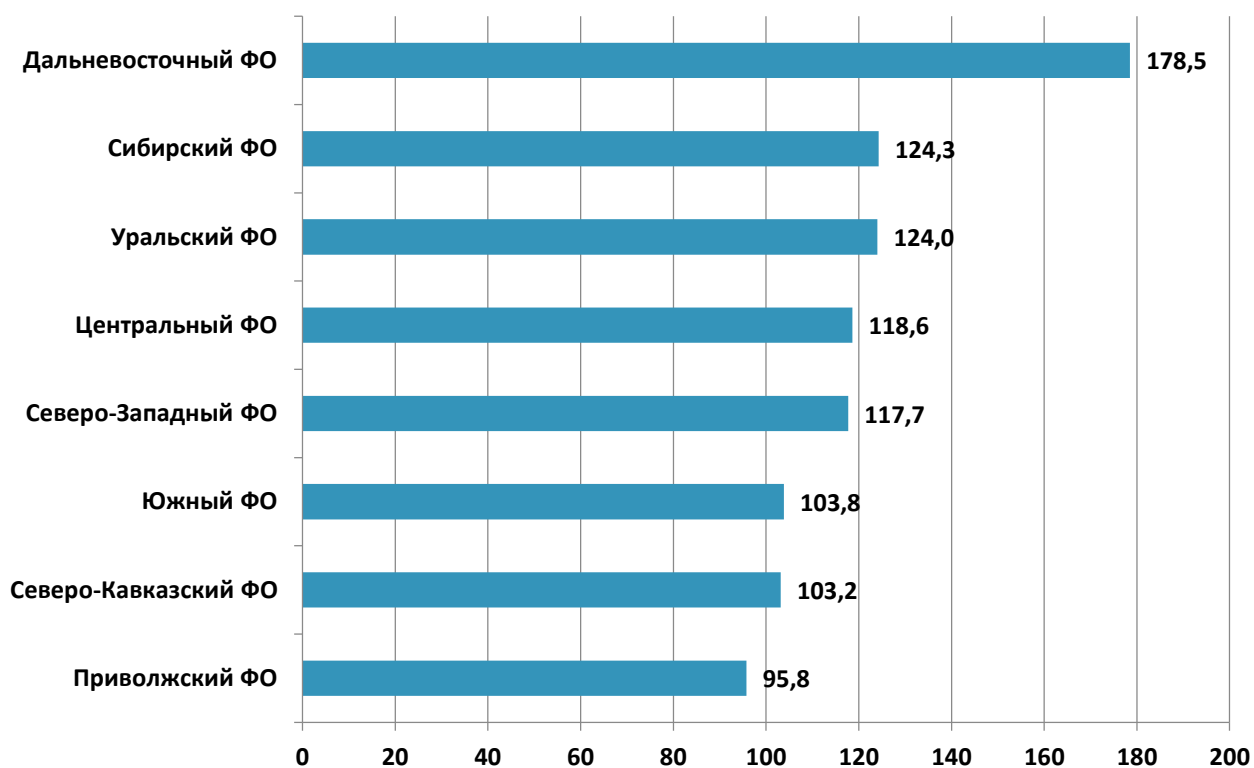
Диаграмма 20. Средние цены на рынке аппаратов орбитальной сварки по Федеральным Округам РФ в 2018 г., руб.
