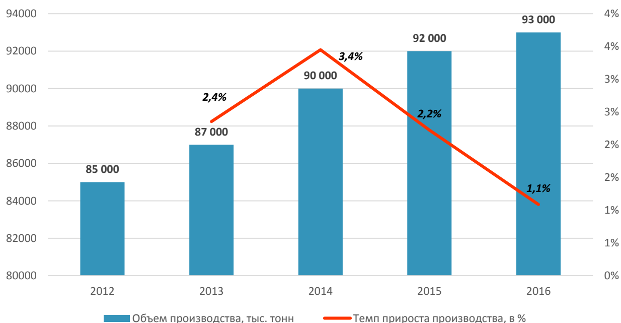
Диаграмма 11. Объем и темп прироста производства блочных стеновых материалов в России в 2012-2016 гг. в натуральном выражении, ..... и %.
