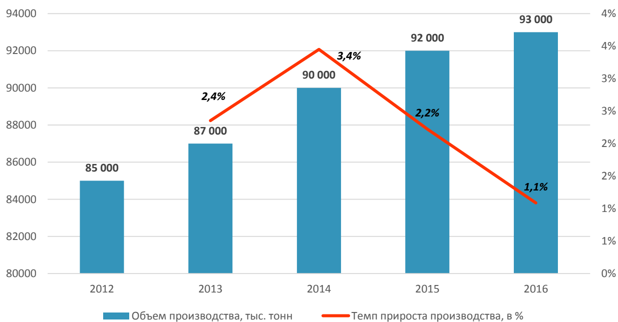
Диаграмма 11. Объем и темп прироста производства блоков из бетона в России в 2012-2016 гг. в натуральном выражении, ..... и %.
