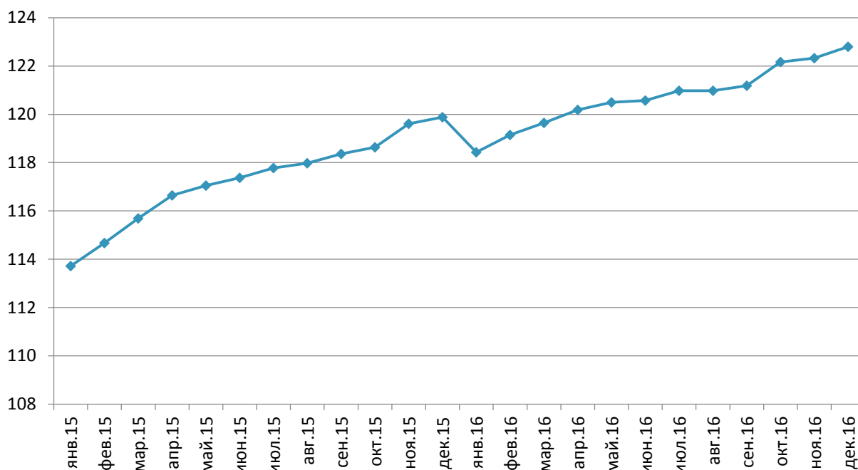
Диаграмма 21. Динамика средних цен на рынке электрических двигателей средней мощности в России в 2015-2016 гг., руб.
