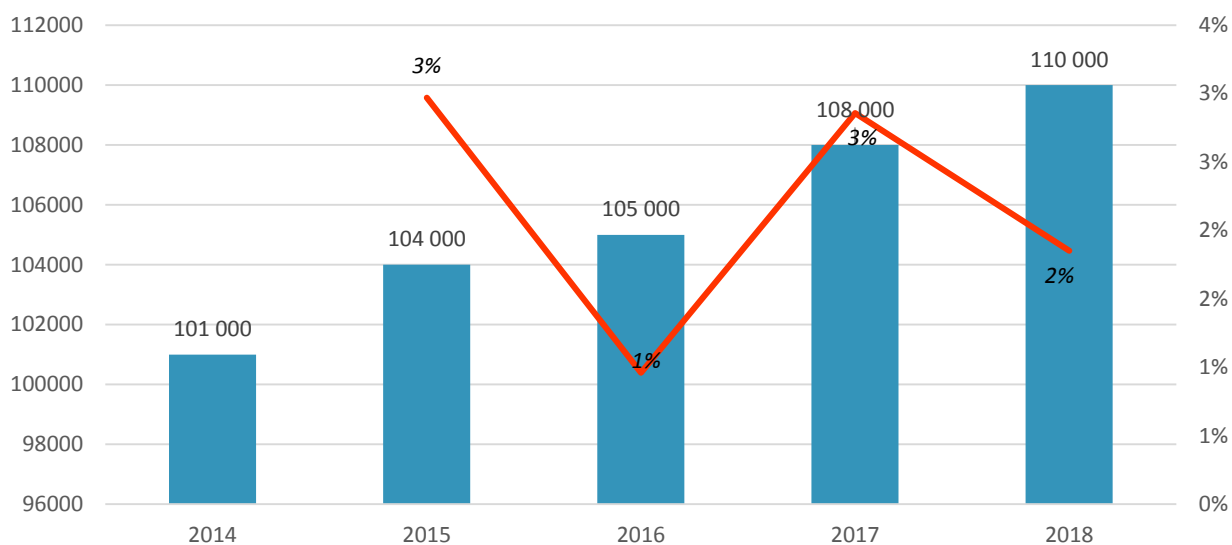
Диаграмма 1. Объем и темп прироста рынка машин для производства металлопластиковых композитных панелей в России в 2014-2018 гг. в натуральном выражении, ..... и %.
