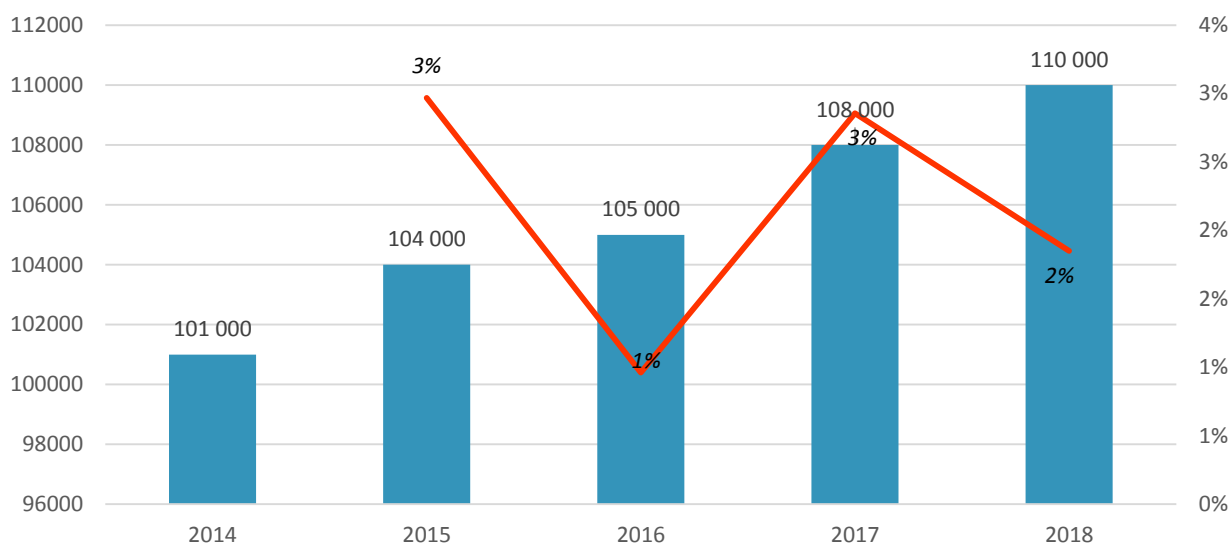
Диаграмма 1. Объем и темп прироста рынка машин для производства труб со стекловолокном в России в 2014-2018 гг. в натуральном выражении, ..... и %.
