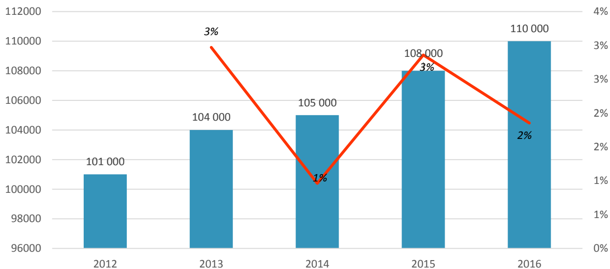
Диаграмма 2. Объем и темп прироста рынка модульных зданий в России в 2012-2016 гг. в стоимостном выражении, $ тыс. и %.
