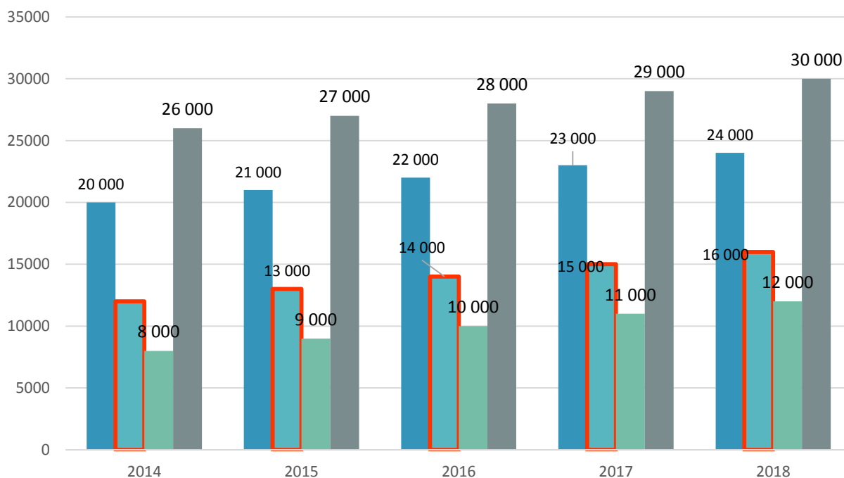
Диаграмма 5. Объём рынка озонаторов для очистки воды в России по сегментам в 2014-2018 гг. в стоимостном выражении, $ тыс.
