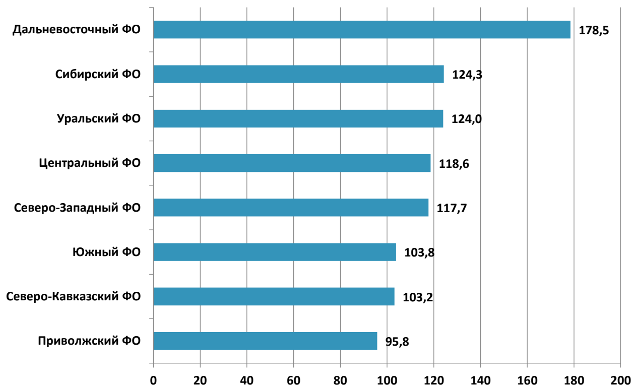
Диаграмма 20. Средние цены на рынке плит газовых по Федеральным Округам РФ в 2016 г., руб.
