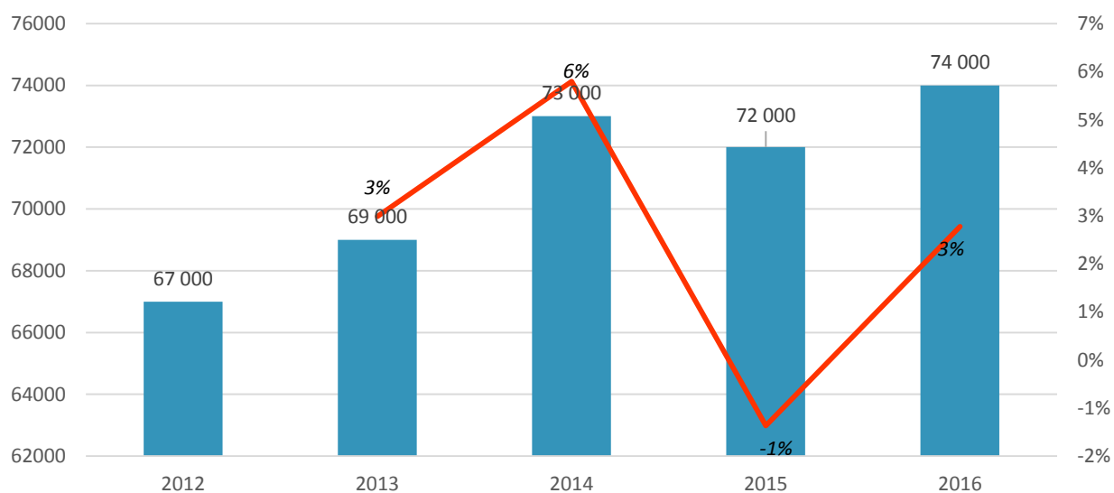
Диаграмма 16. Объём и темп прироста производства Сегмента 1 «.....» рынка станков токарно-винторезных в России в 2014-2018 гг. в натуральном выражении, ..... и %.
